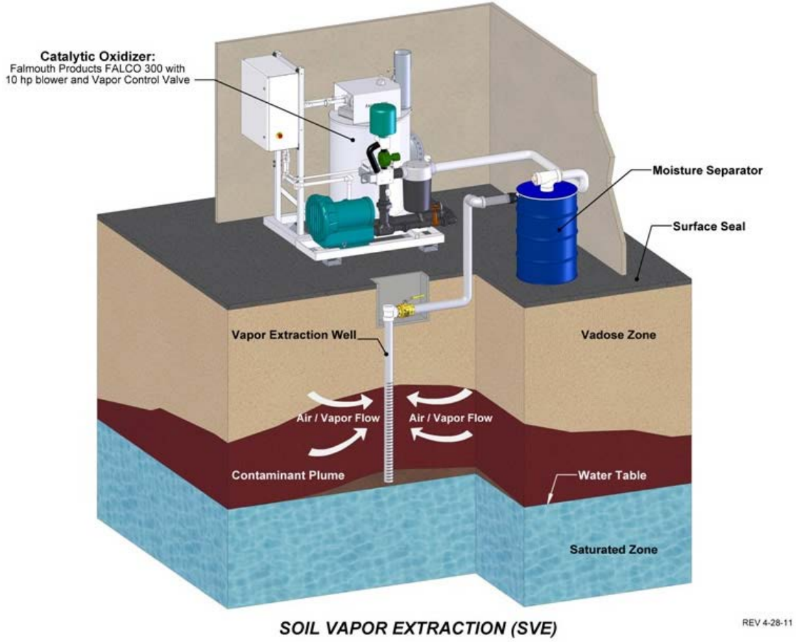
Şekil 1.1- SVE –Toprak Gazı Şeması.
