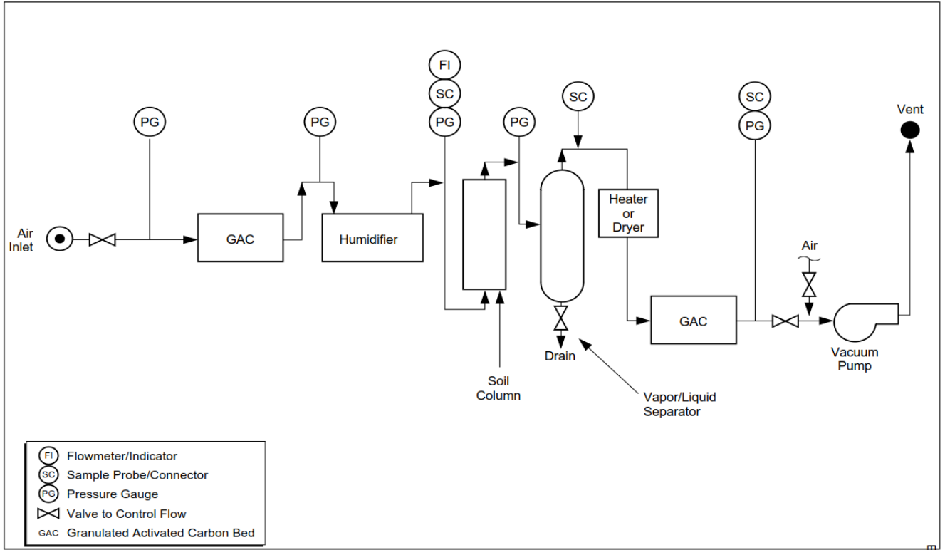
Şekil 3.3- Bir Kolon test Cihazının Şeması
