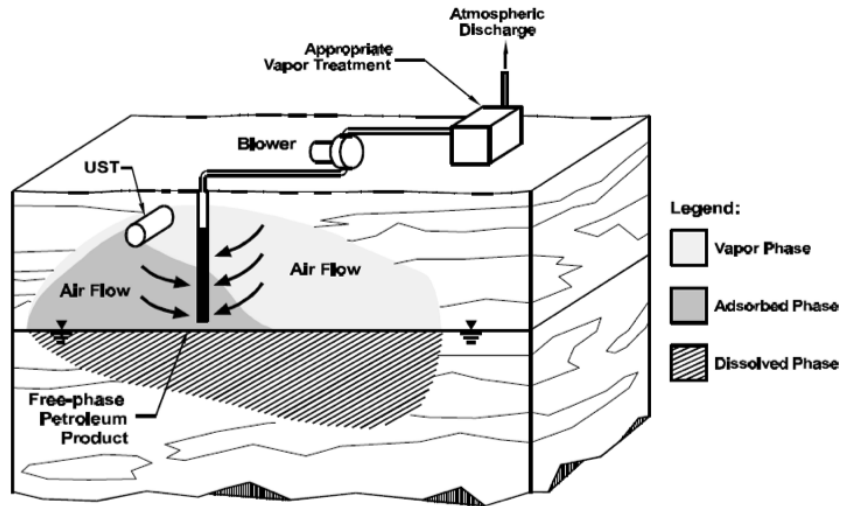
Şekil 4.9- Bir fan ile oluşturulmuş şema
