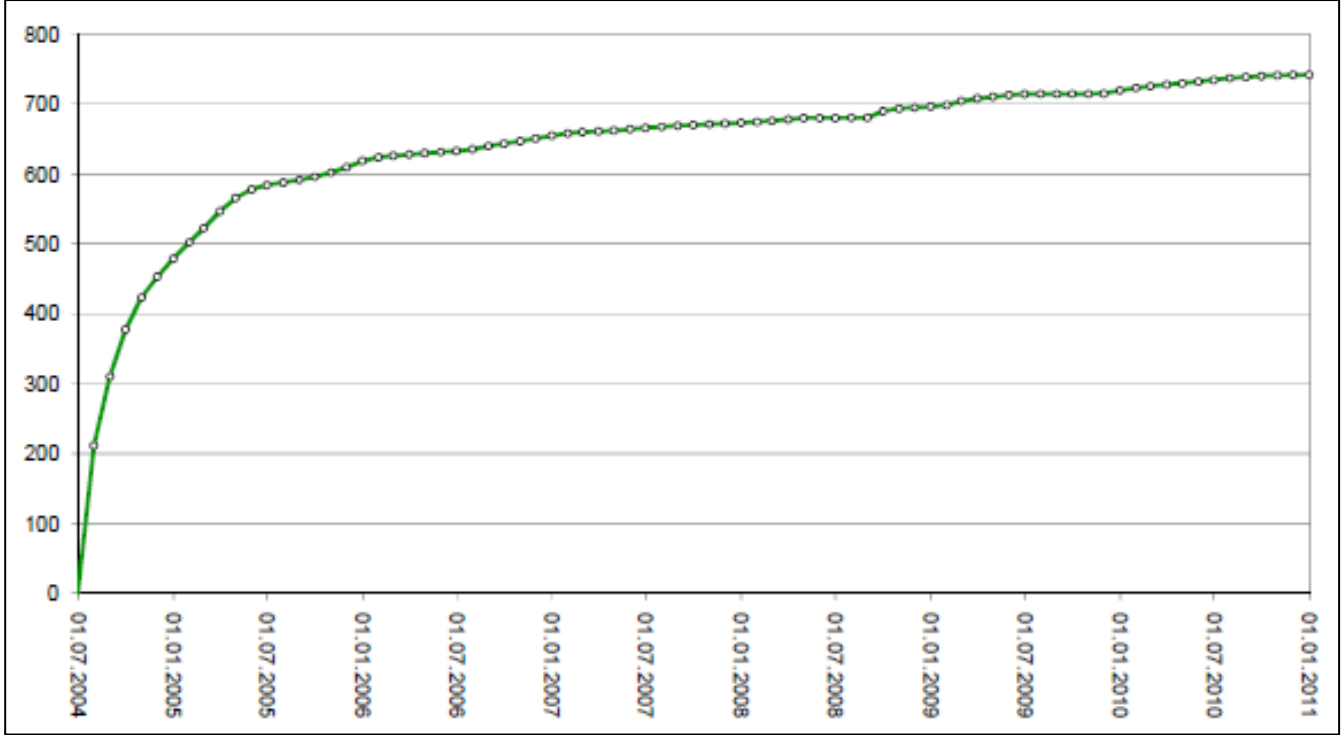
Şekil 5.2 – Kirlenici kütlesi giderimindeki eğilimler (TGE): kg PCE (toplam zaman)
