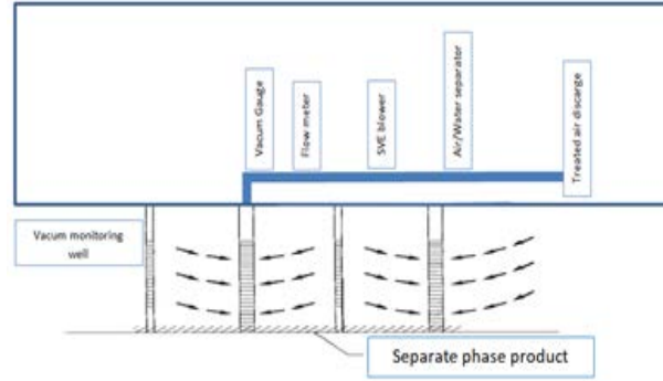
Şekil 2.1- Toprak Buharı/Gazı Ekstraksiyonu (SVE) Tesisinin Bşleşenleri
