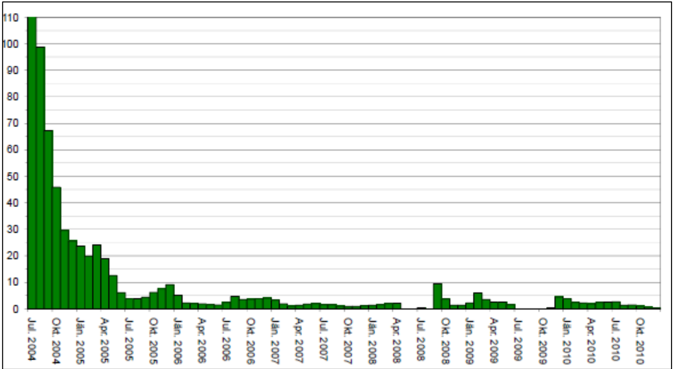
Şekil 5.1 – Kirletici kütlesi giderimindeki eğilimler (TGE): kg PCE/gün
