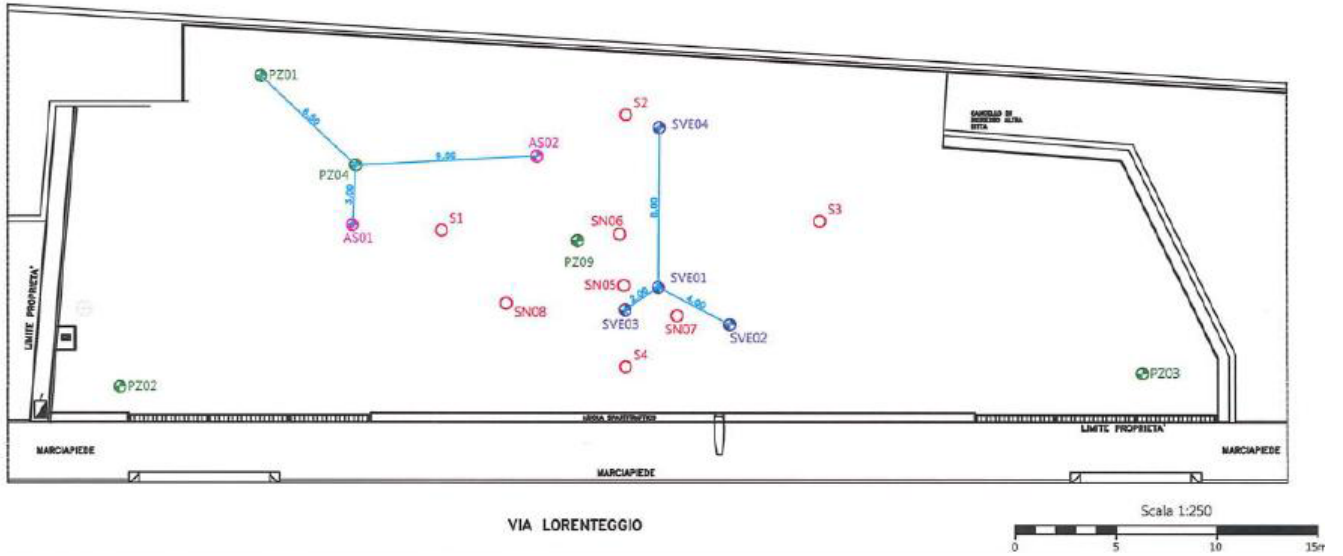
Şekil 4.5- TGE izleme noktasının 120° 'sinde tipik bir konuşlandırma (Confalonieri vd., bkz Ek1)
