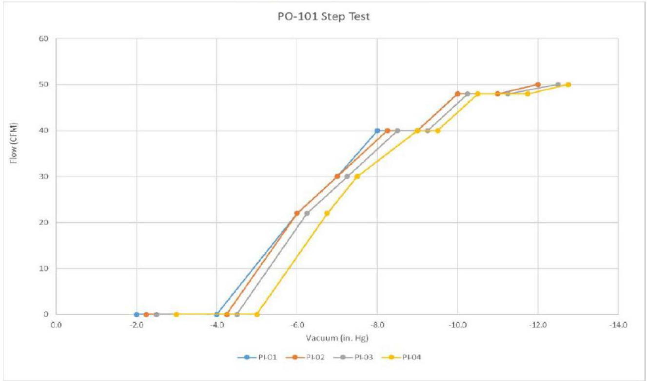
Şekil 4.7- TGE artan vakum basamağı testi örneği (Menozzi vd., bkz. Ek1)
