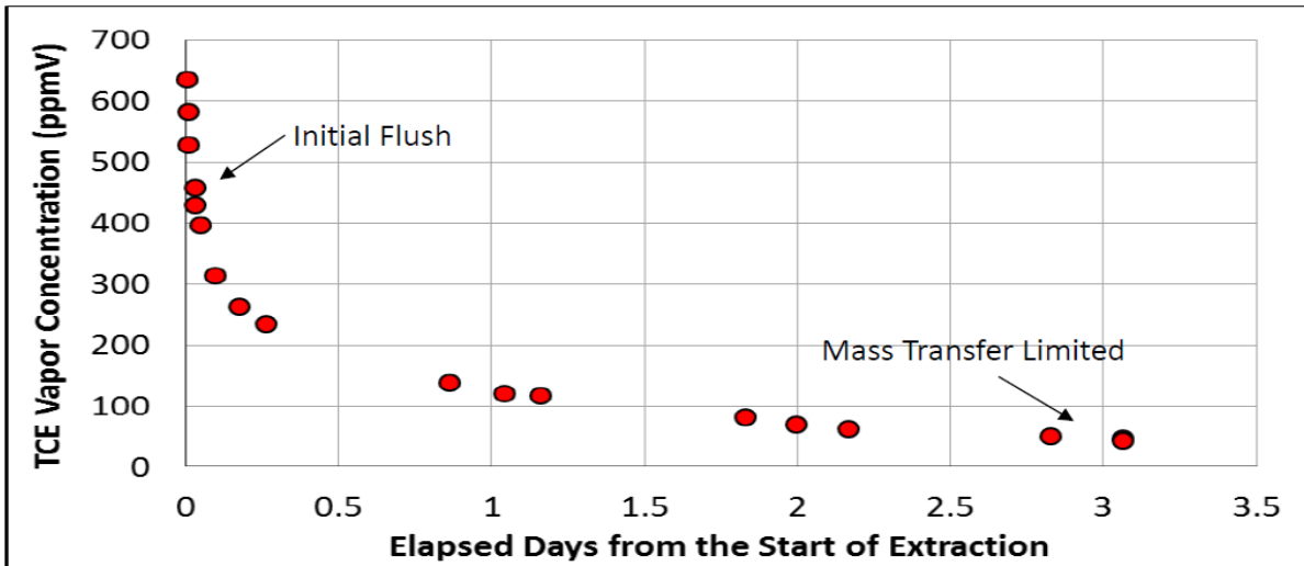
Şekil 4.2- TGE pilot testinden örnek gaz konsantrasyon verisi
