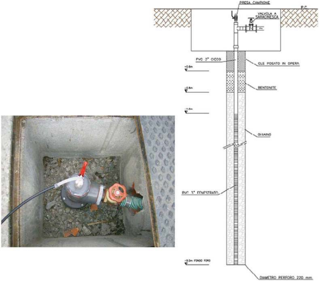
Şekil 4.8- Yuva Sonda Kurulum Örneği (Trezzi vd., bkz. Ek1)
