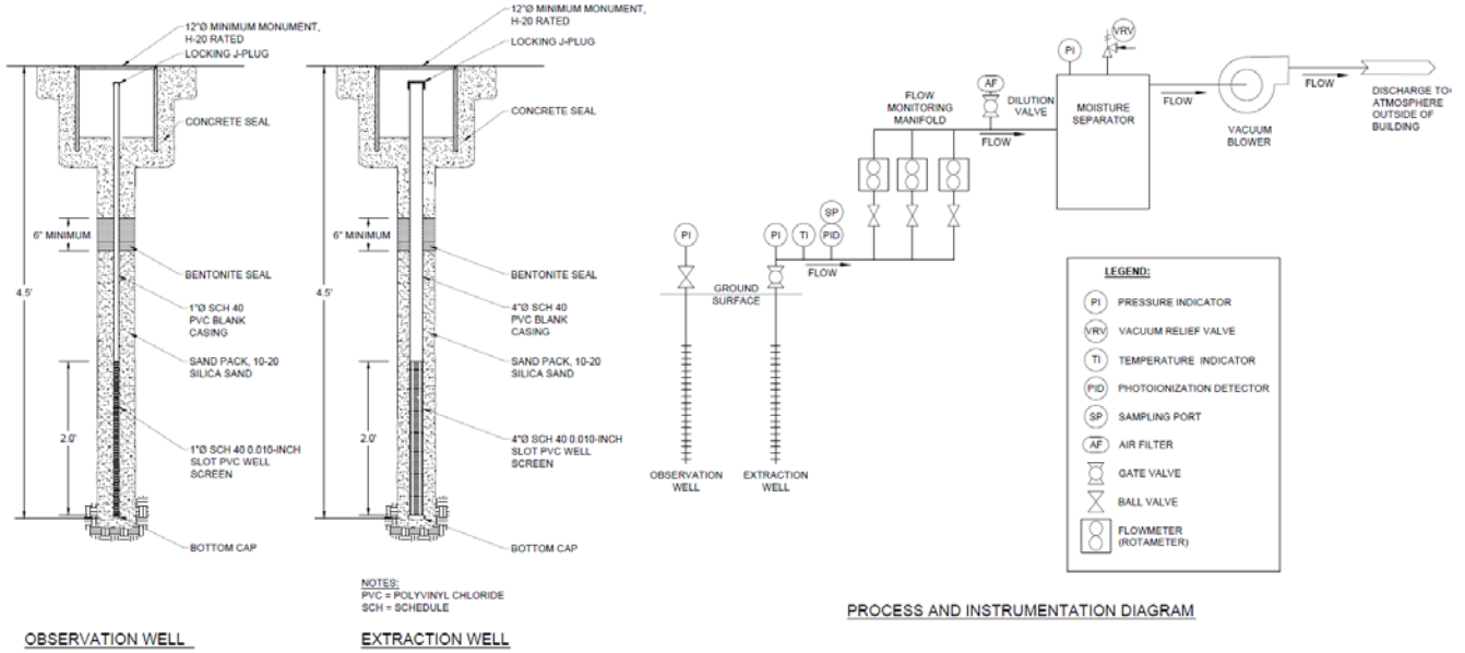
Şekil 4.4- Örnek proses ve cihaz diyagramı (Farallon Consulting)
