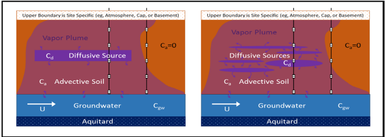
Sekil 4.3- Difüzyon sınırlı kütle transferi ve tipik toprak gazı izleme noktaları için kavramsallaştırılmış senaryolar
