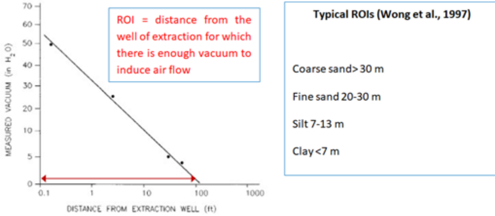
Şekil 2.4- Etki Yarıçapı
