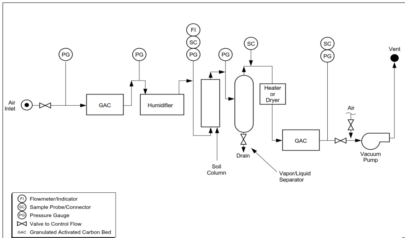
Slika 3.3- Diagram kolonske preizkusne naprave
