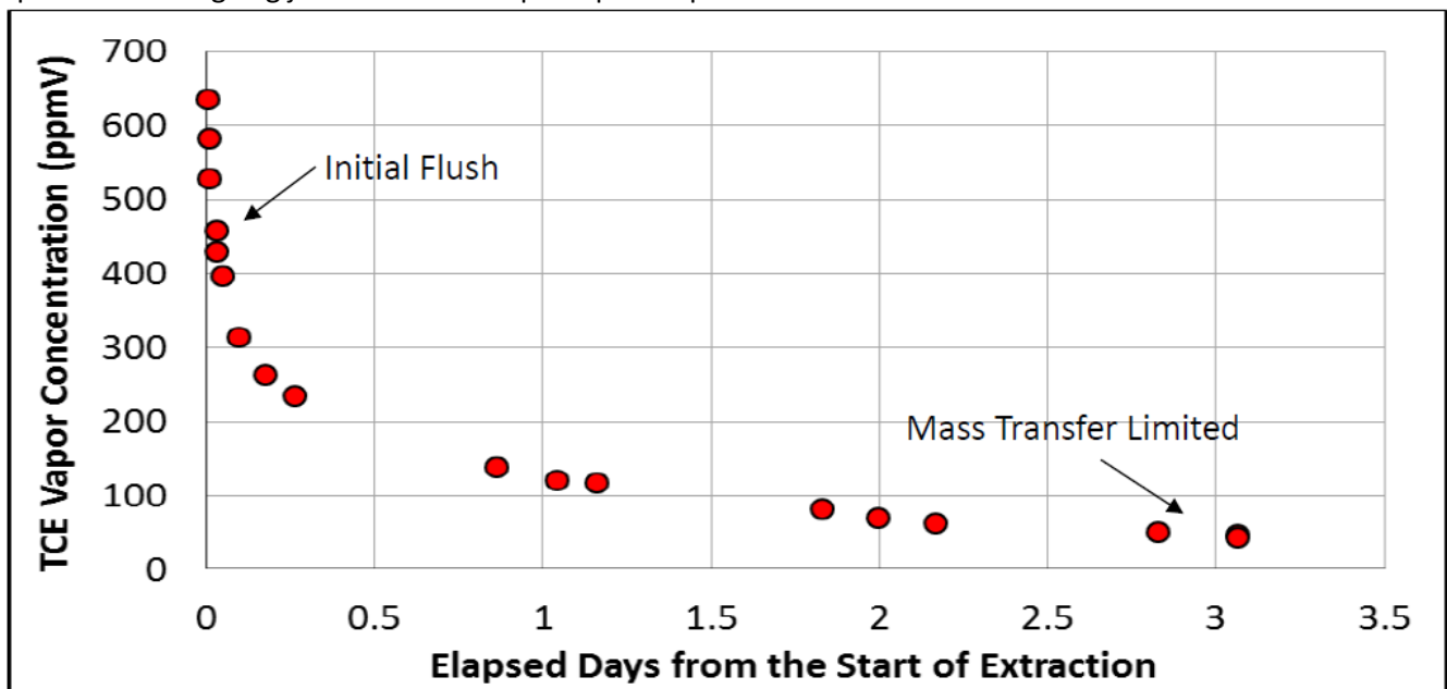
Slika 4.2- Primer podatkov o koncentraciji hlapov iz pilotnega preizkusa SVE
