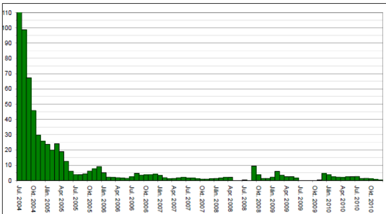
Slika 5.1 – Trendi odstranjevanja mase kontaminantov (SVE): kg PCE/day
