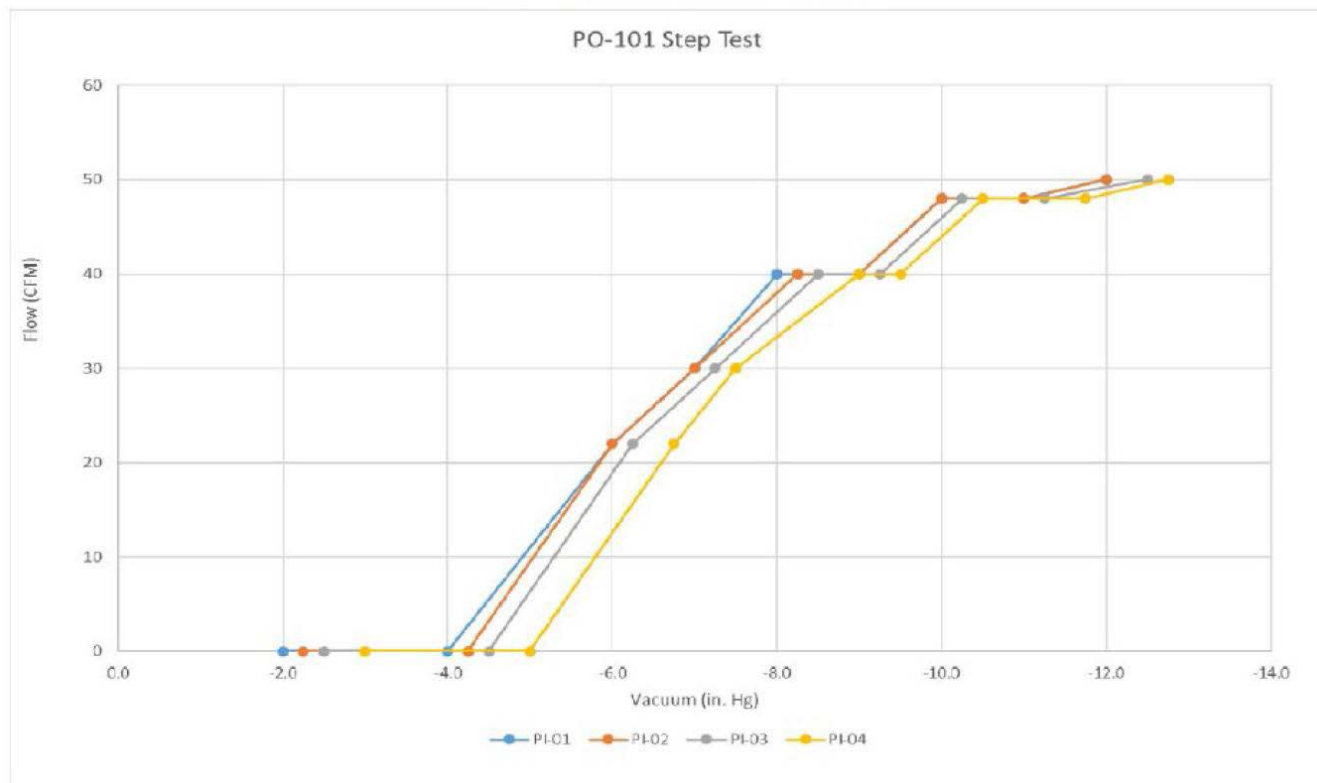
Slika 4.7- Primer preizkusa stopnje povečanja vakuuma SVE (Menozi et al., see Annex1)
