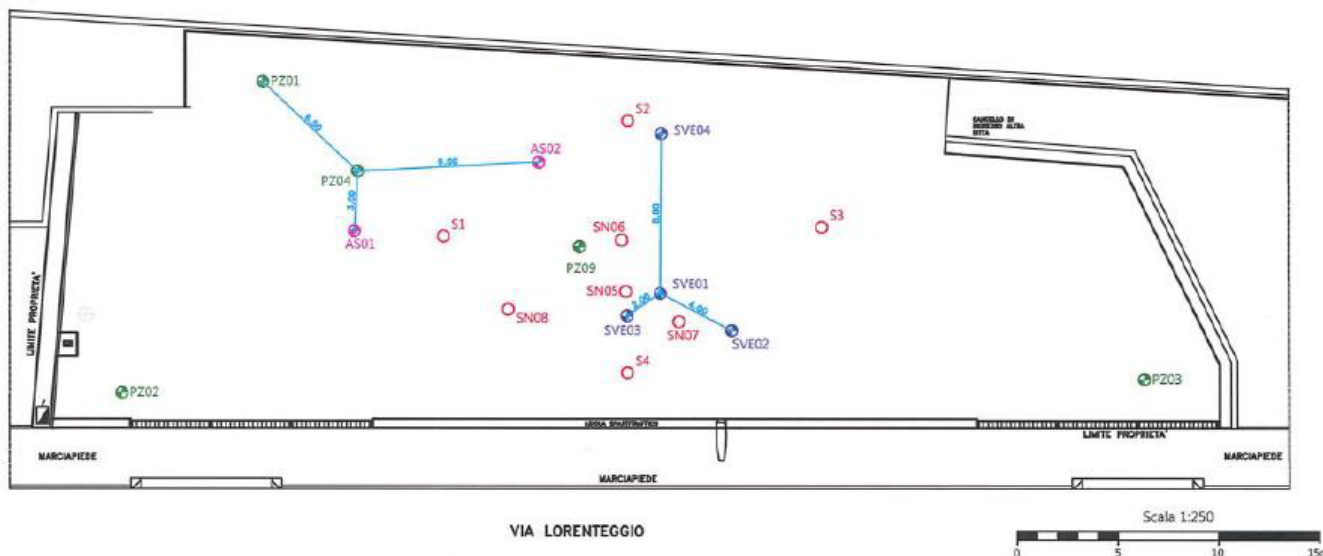
Slika 4.5- Tipična postavitev pri 120° monitorni točki SVE (Confalonieri et al., Annex1)
