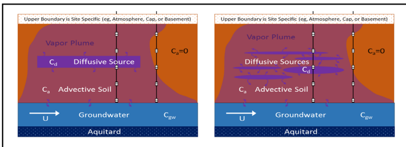
Slika 4.3- Konceptualizirani scenariji za difuzijsko omejen prenos mase in tipične točke spremljanja plinov v tleh
