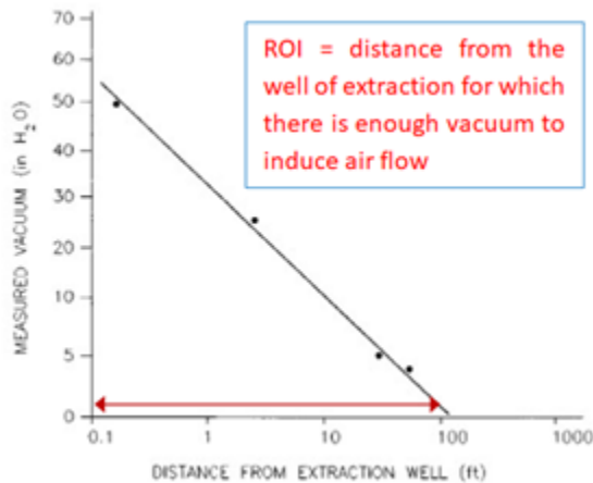
Slika 2.4- Vplivni radij
