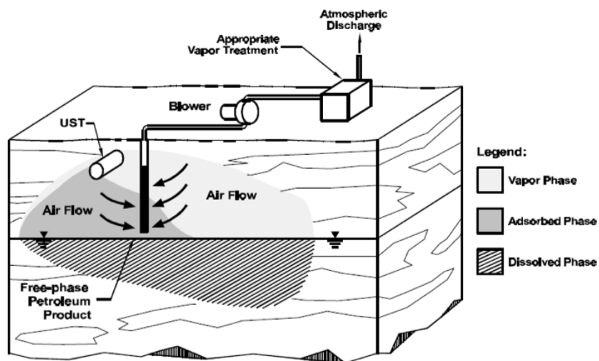
Slika 4.9- Shema z enim puhalom
