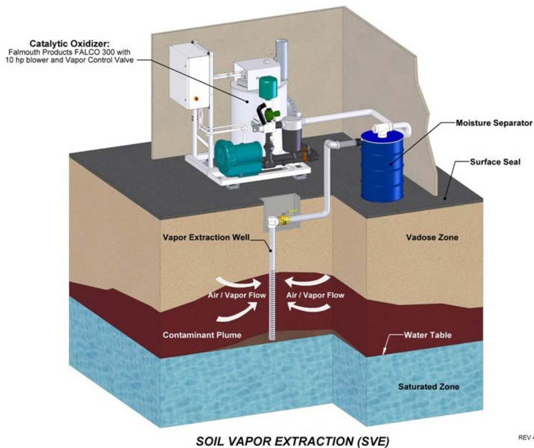
Slika 1.1- shema delovanja SVE.
