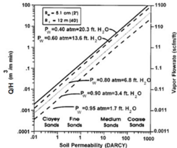
Slika 2. Hitrost ekstrakcije
