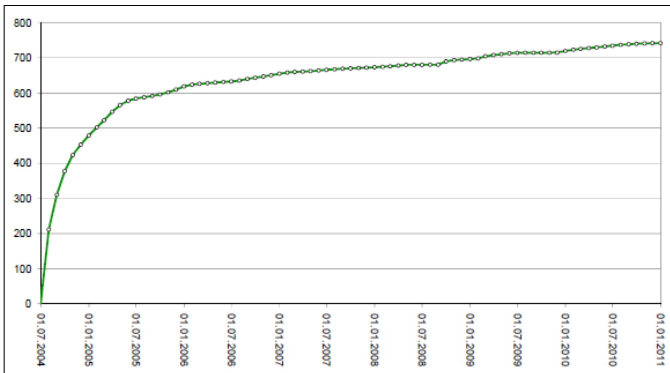
Slika 5.2 – Trendi odstranjevanja mase kontaminantov (SVE): kg PCE (celotno skozi čas)
