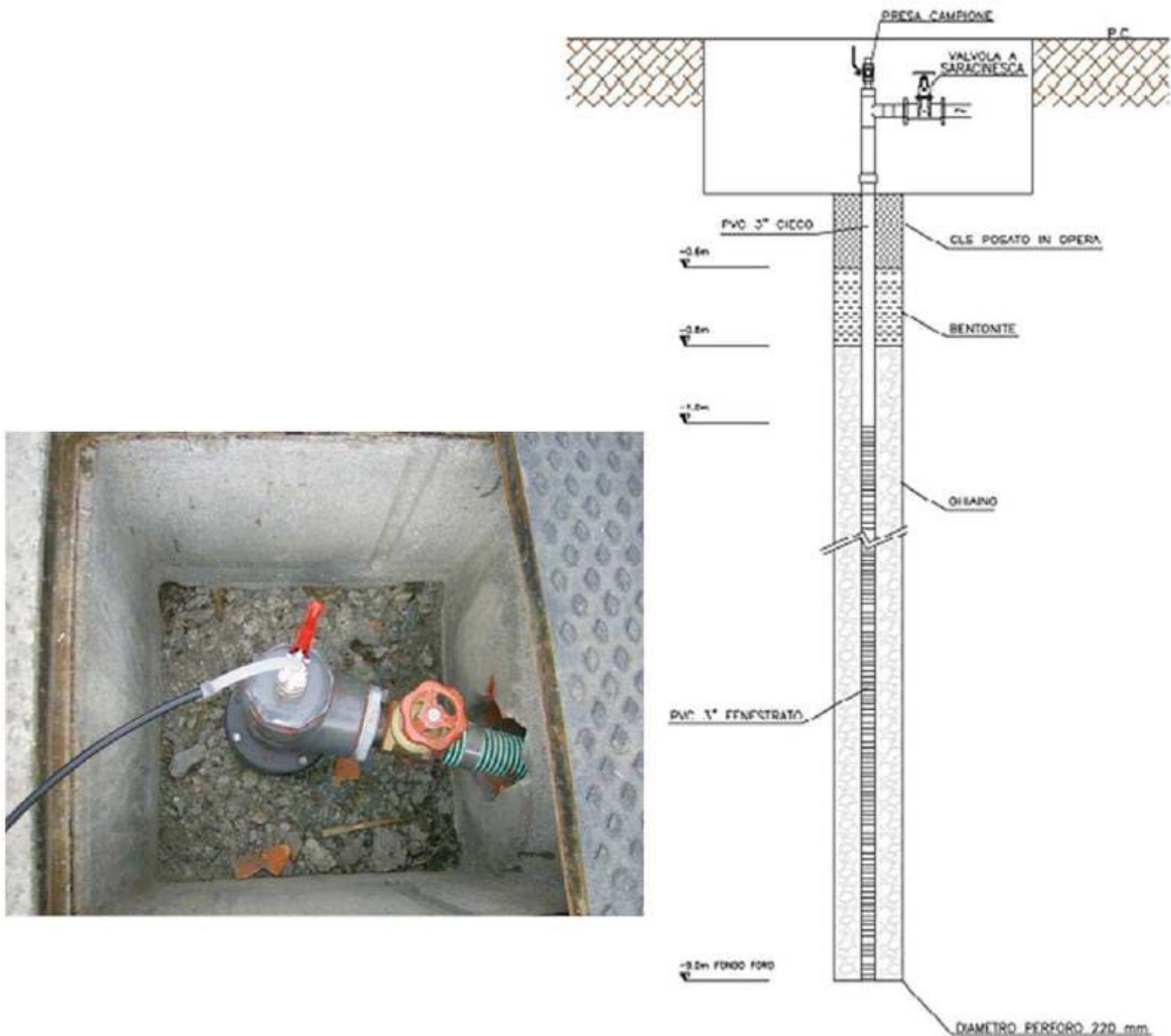
Slika 4.8- Primer namestitve Nesty sonde (Trezzi et al., see Annex1)
