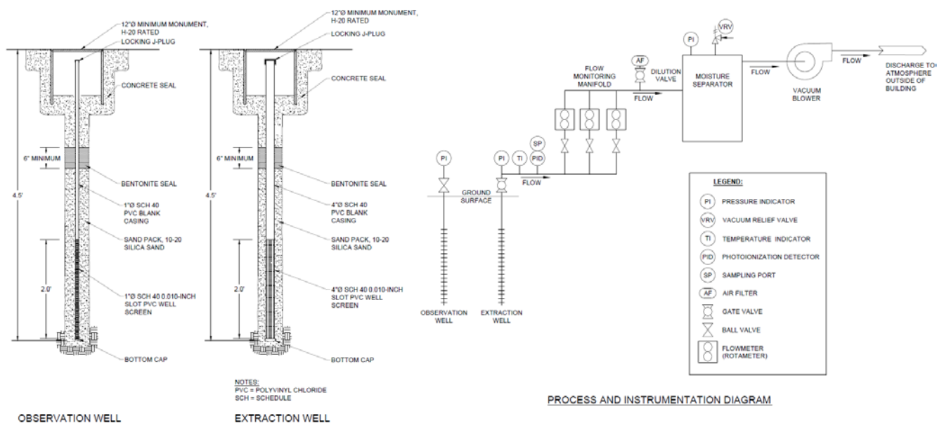
Slika 4.4- Primer diagrama procesa in instrumentacije (Farallon Consulting)
