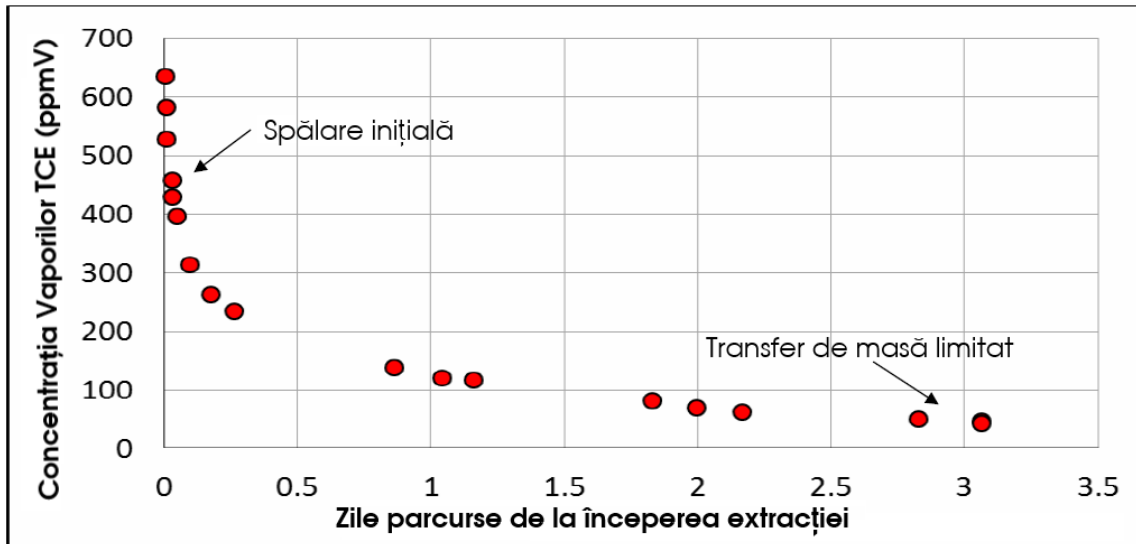
Figura 4.2- Exemplu de date privind concentrația de vapori de la un test pilot SVE
