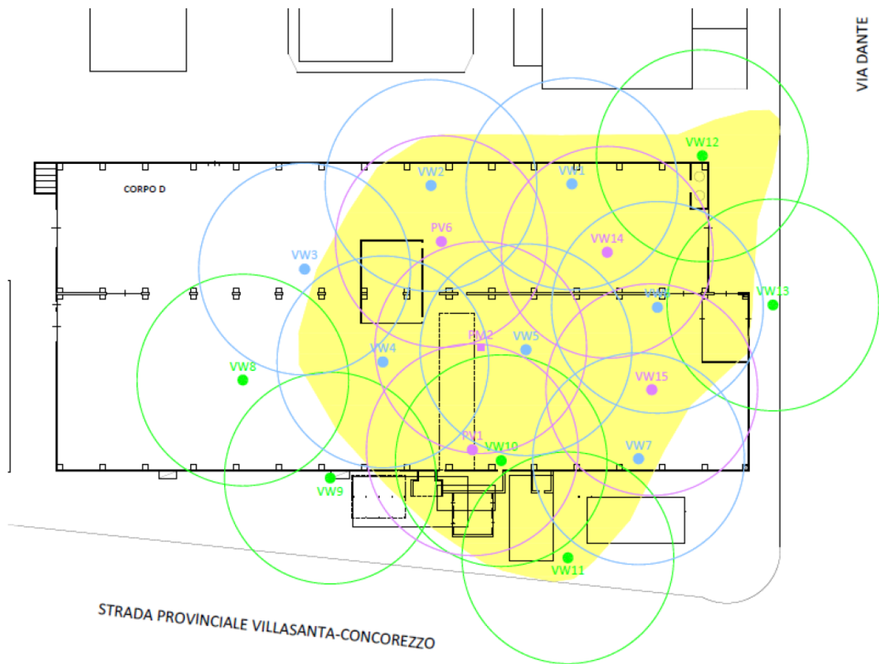
Figura 4.1- Raza de influență după Testul pilot (Confalonieri et al., see Annex1)
