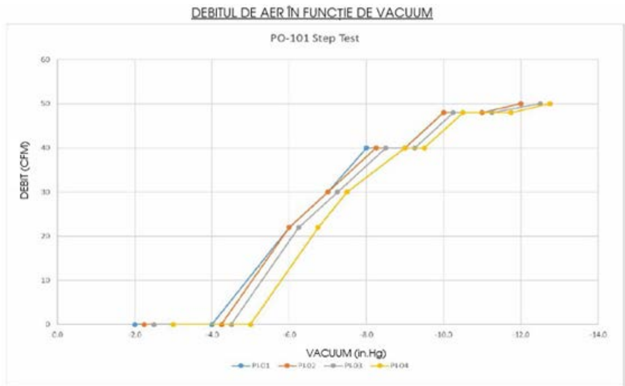
Figure 4.7- Exemplu de test de creștere a vidului în trepte SVE (Menozzi et al., vezi Anexa 1)
