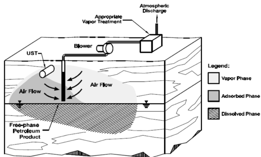
Figura 4.9- Esquema com um ventilador
