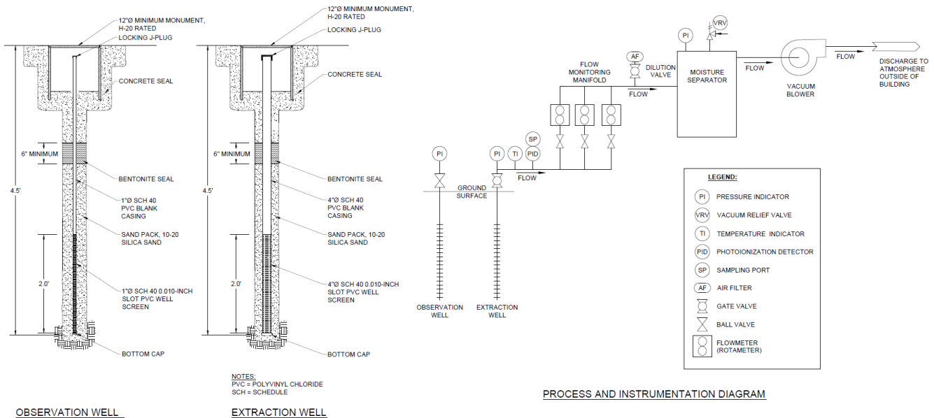
Figura 4.4. Exemplo de diagrama de processo e instrumentação (Farallon Consulting).
