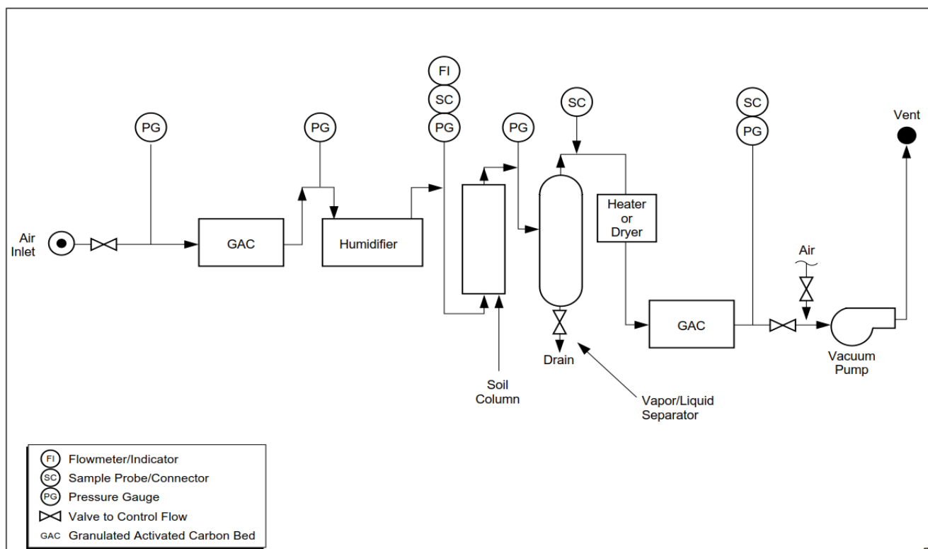
Figura 3.3- Diagrama para ensaio em coluna
