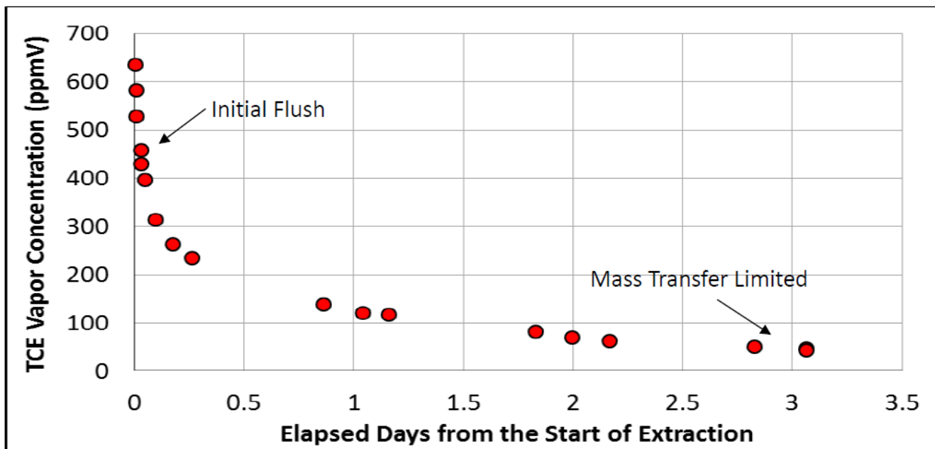
Figure 4.2- Exemplo de dados de concentração de vapor de um teste piloto SVE
