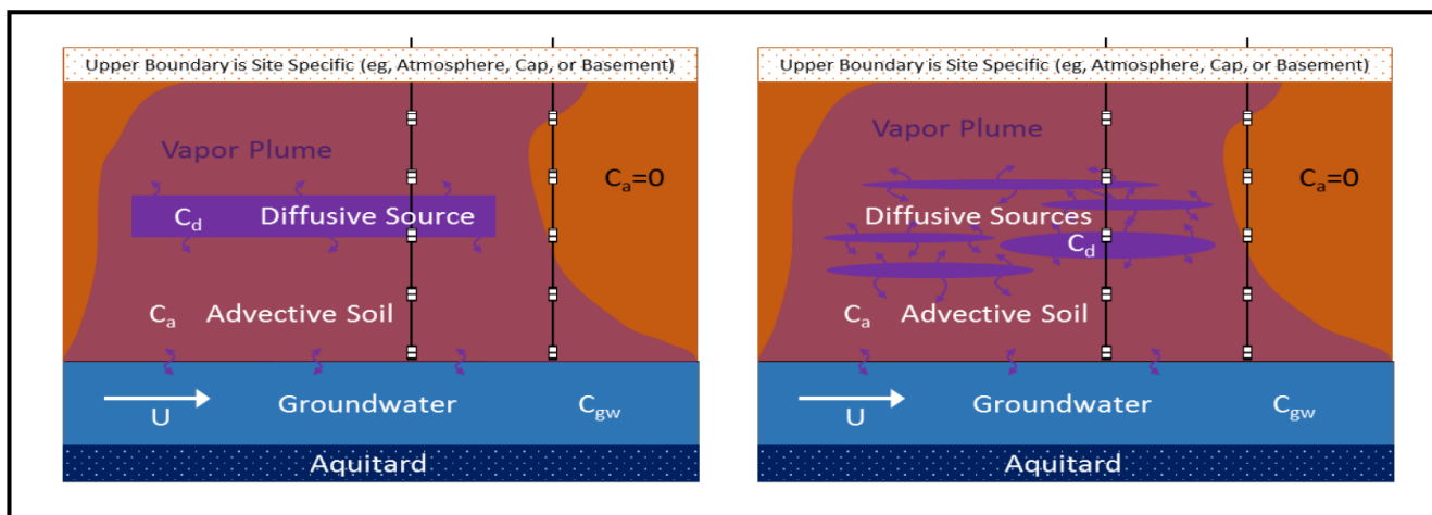
Figura 4.3- Cenários conceituais para a transferência de massa limitada por difusão e pontos típicos de monitorização de gás do solo
