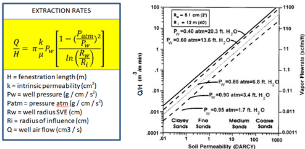
Figura 2.6 Taxas de extração
