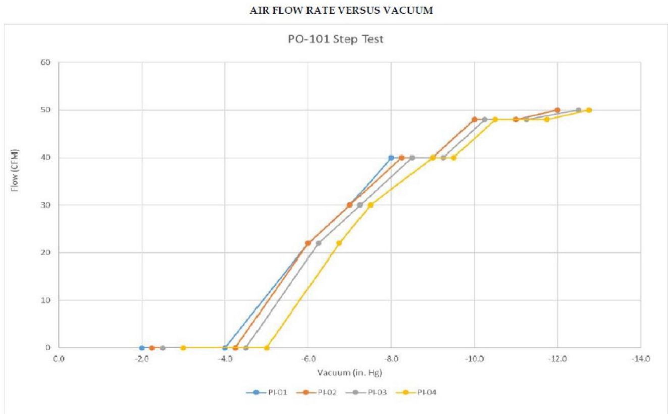
Figura 4.7- Exemplo de teste de etapas crescentes de vácuo SVE (Menzio et al., ver Anexo 1)
