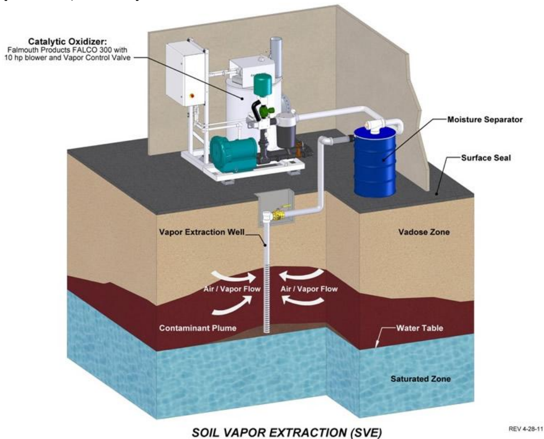
Figura 1.1- Esquema da SVE
