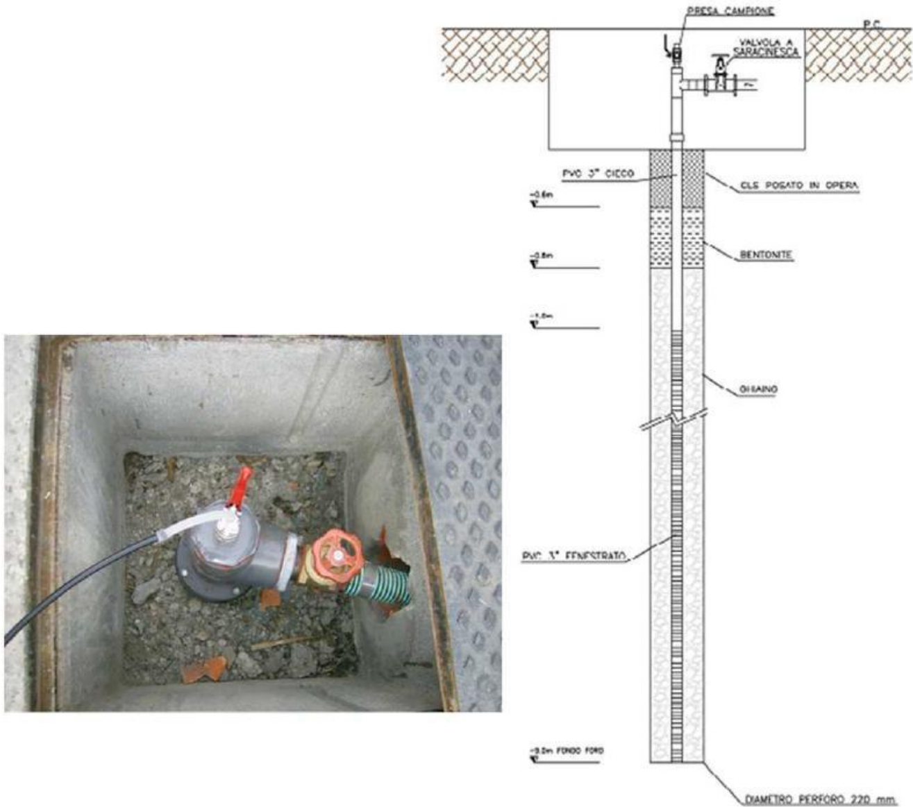
Figura 4.8 - Exemplo de instalação da Sonda Nesty (Trezzi et al., ver Anexo 1)
