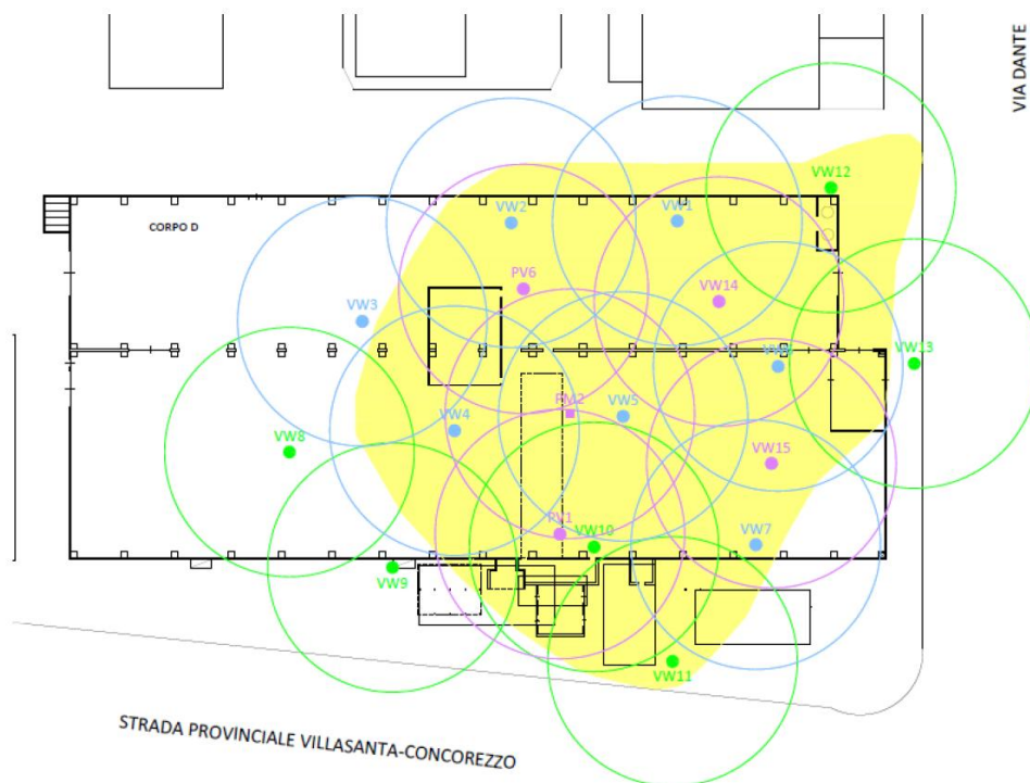
Figura 4.1- Raio de influência após o teste piloto (Confalonieri et al., ver Anexo 1)
