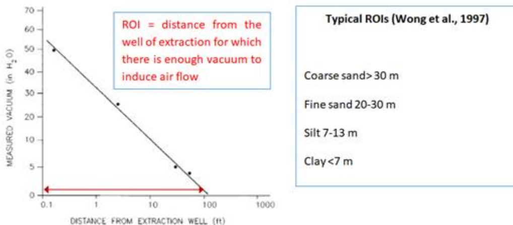
Figura 2.4- Raio de influência
