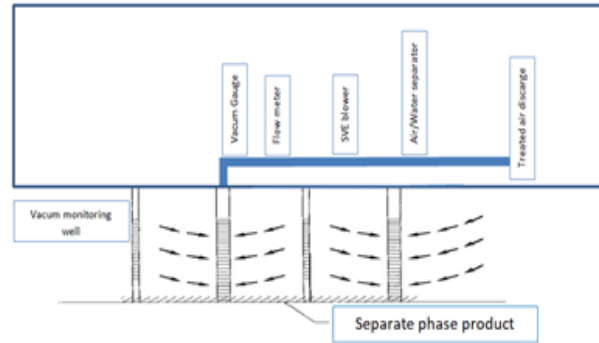
Figura 2.1- Componentes do sistema SVE
