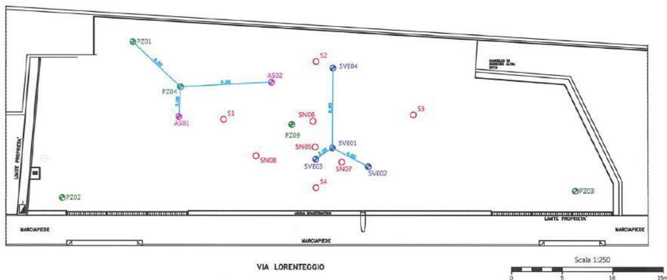
Figura 4.5- Posicionamento típico a 120° do ponto de monitorização SVE (Confalonieri et al., ver Anexo 1)
