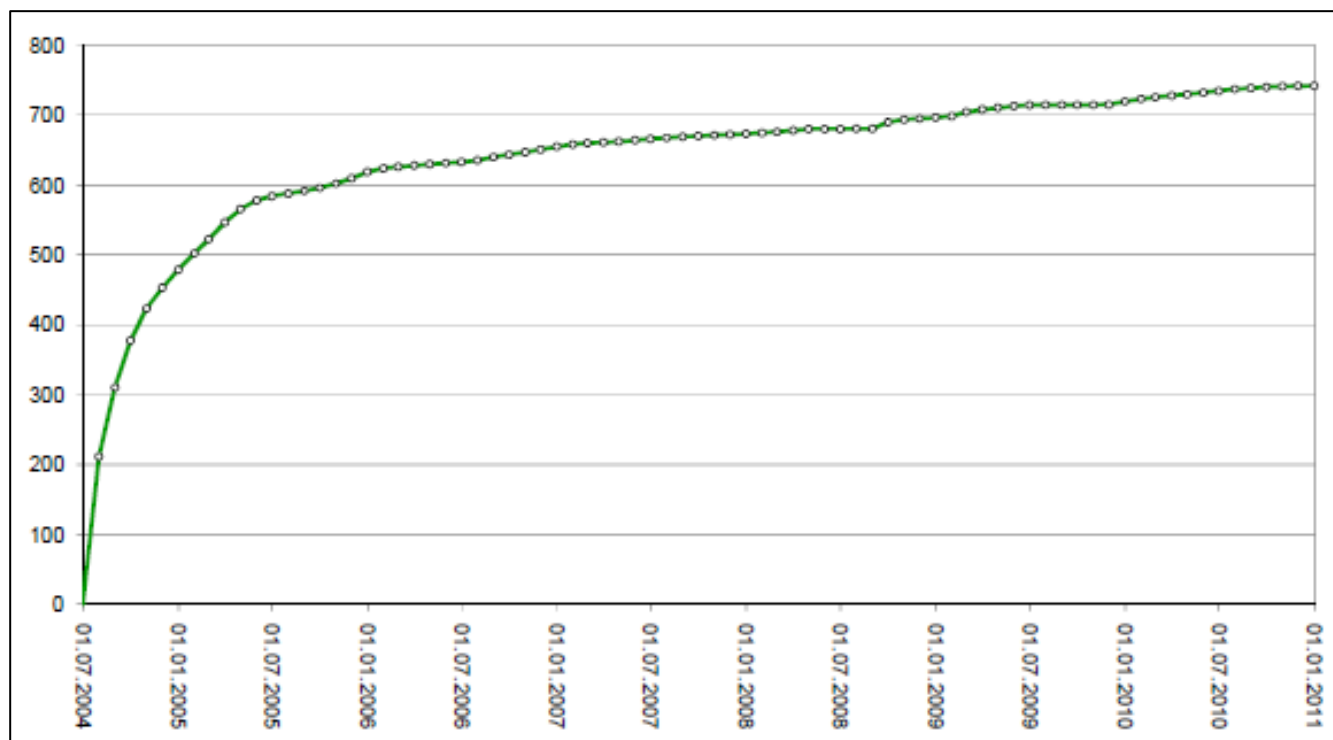
Figura 5.2 – Tendências na remoção de massa contaminante (SVE): kg PCE (total ao longo do tempo)
