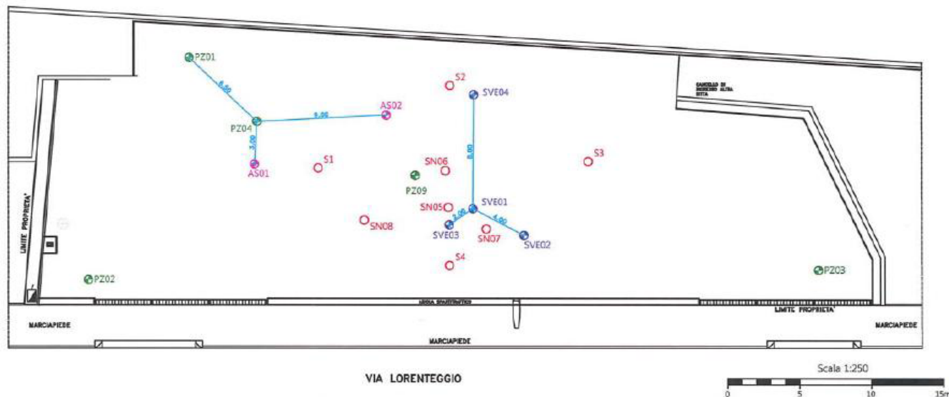
Rysunek 4.5- Pozycjonowanie pod kątem 120^\circ punktów monitorowania SVE (Confalonieri et al., patrz Załącznik 1)
