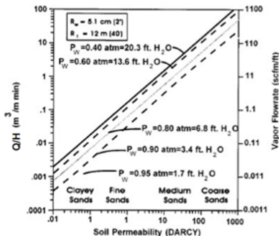
Rysunek 2.6 Wydajność
