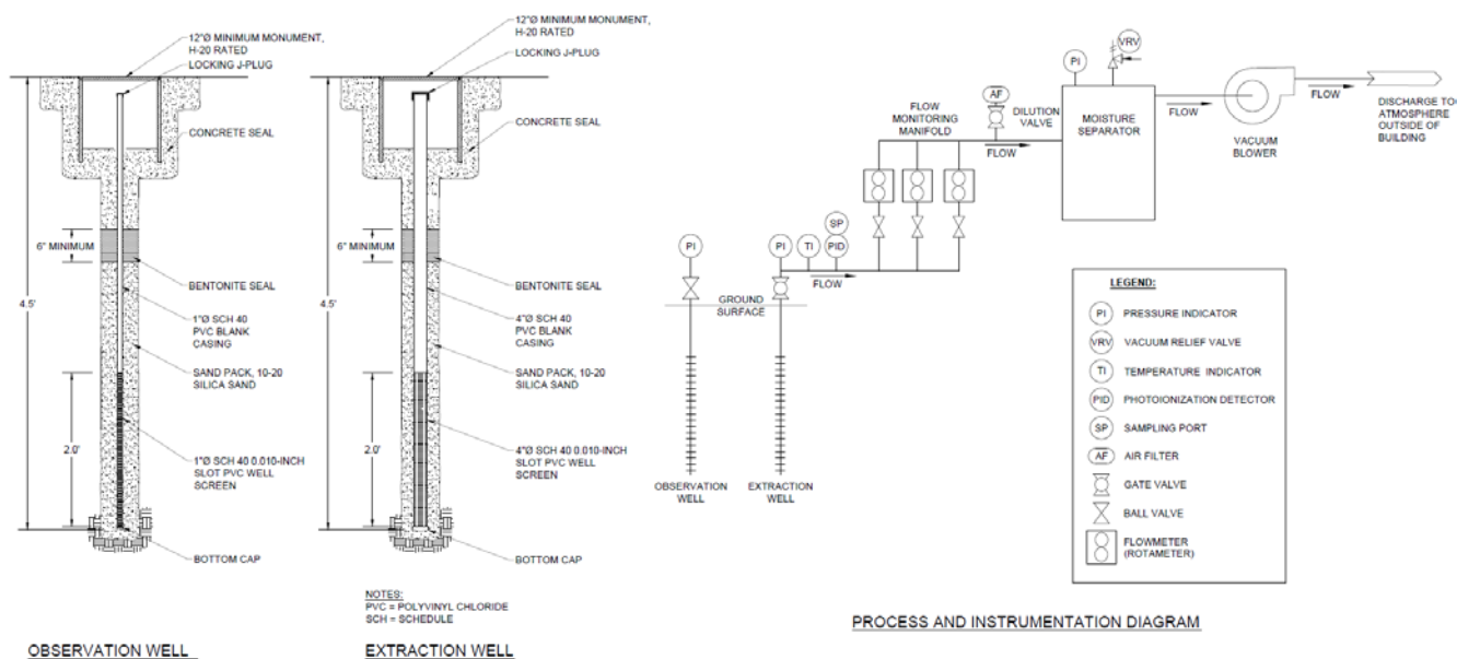
Rysunek 4.4- Przykład procesu i oprzyrządowania (Farallon Consulting)
