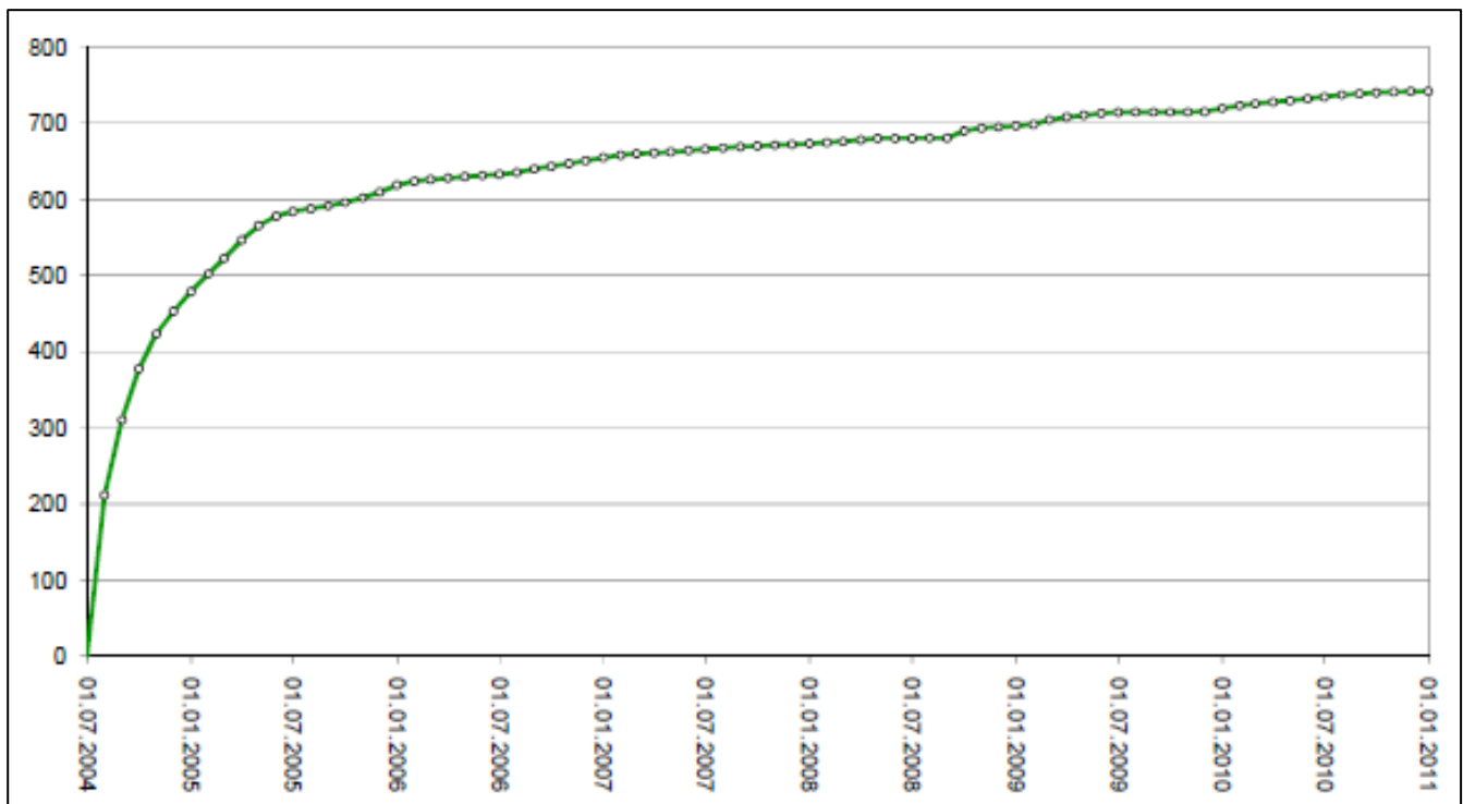
Rysunek 5.2 – Trend usuwania masy zanieczyszczeń (SVE): kg PCE (suma w czasie)
