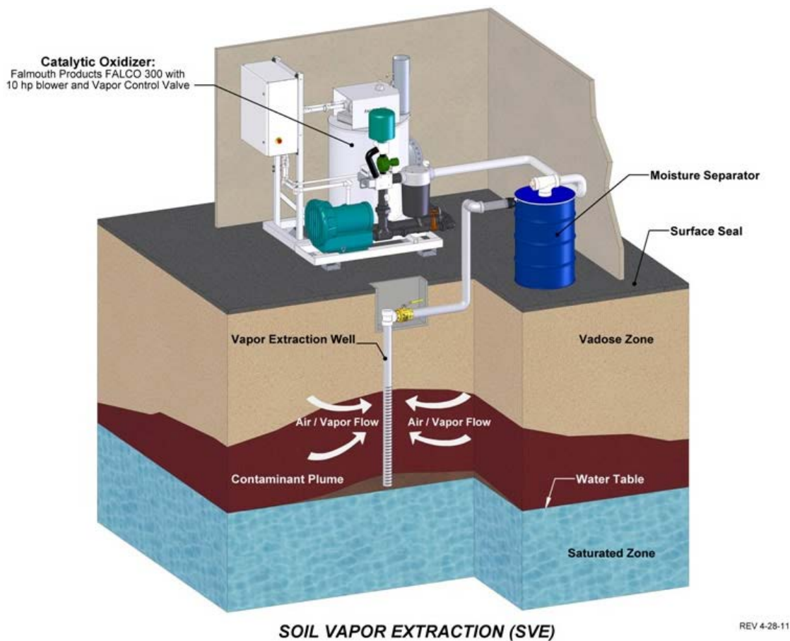
Rysunek 1.1- Schemat procesu SVE
