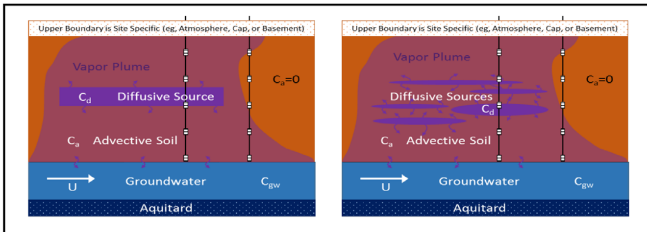
Rysunek 4.3- Konceptyjne scenariusze ograniczonego dyfuzyjnie przenoszenia masy i typowe punkty monitorowania powietrza gruntowego
