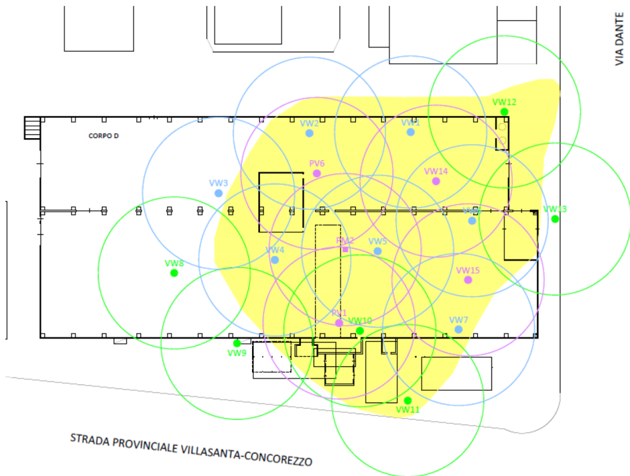
Rysunek 4.1- Promień oddziaływania po wykonaniu testu pilotażowego (Confalonieri et al., patrz załącznik 1)
