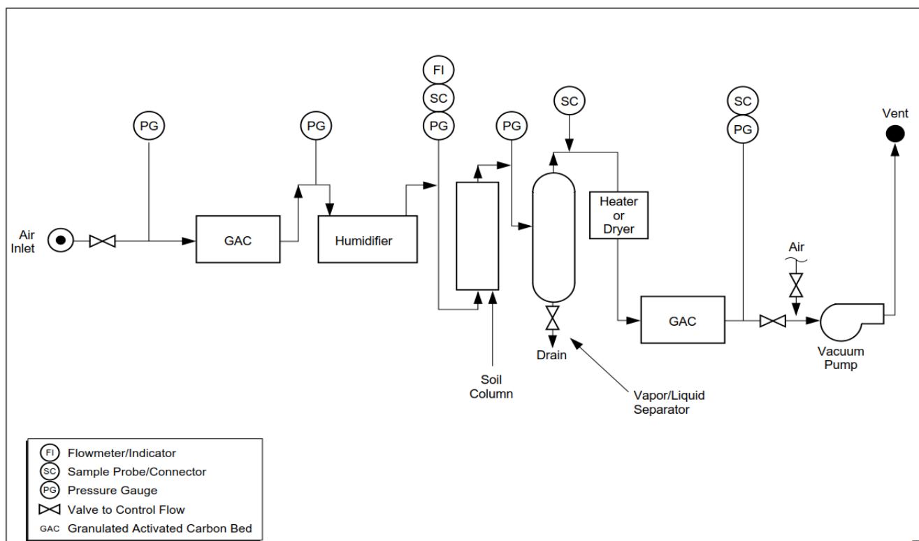
Rysunek 3.3- Schemat kolumnowego aparatu badawczego
