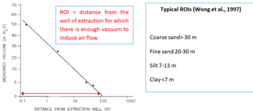
Rysunek 2.4 – Promień oddziaływania
