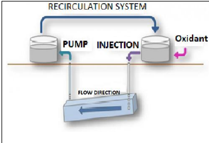
Figura 2.2- Esquema do Sistema de recirculação
