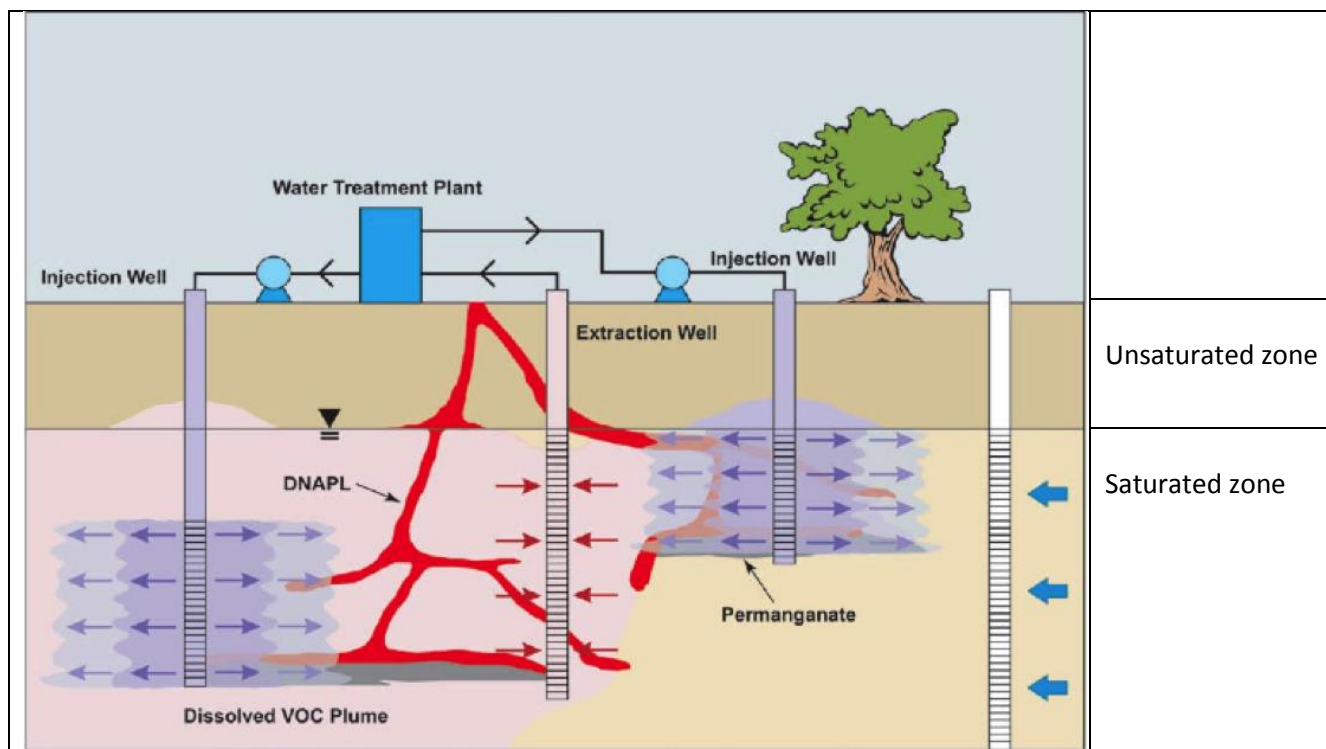
Figura 2.1- Esquema ISCO
