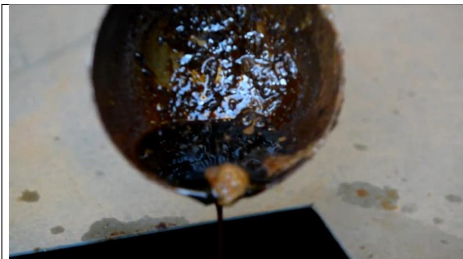
Figura 2.6- DNAPL
