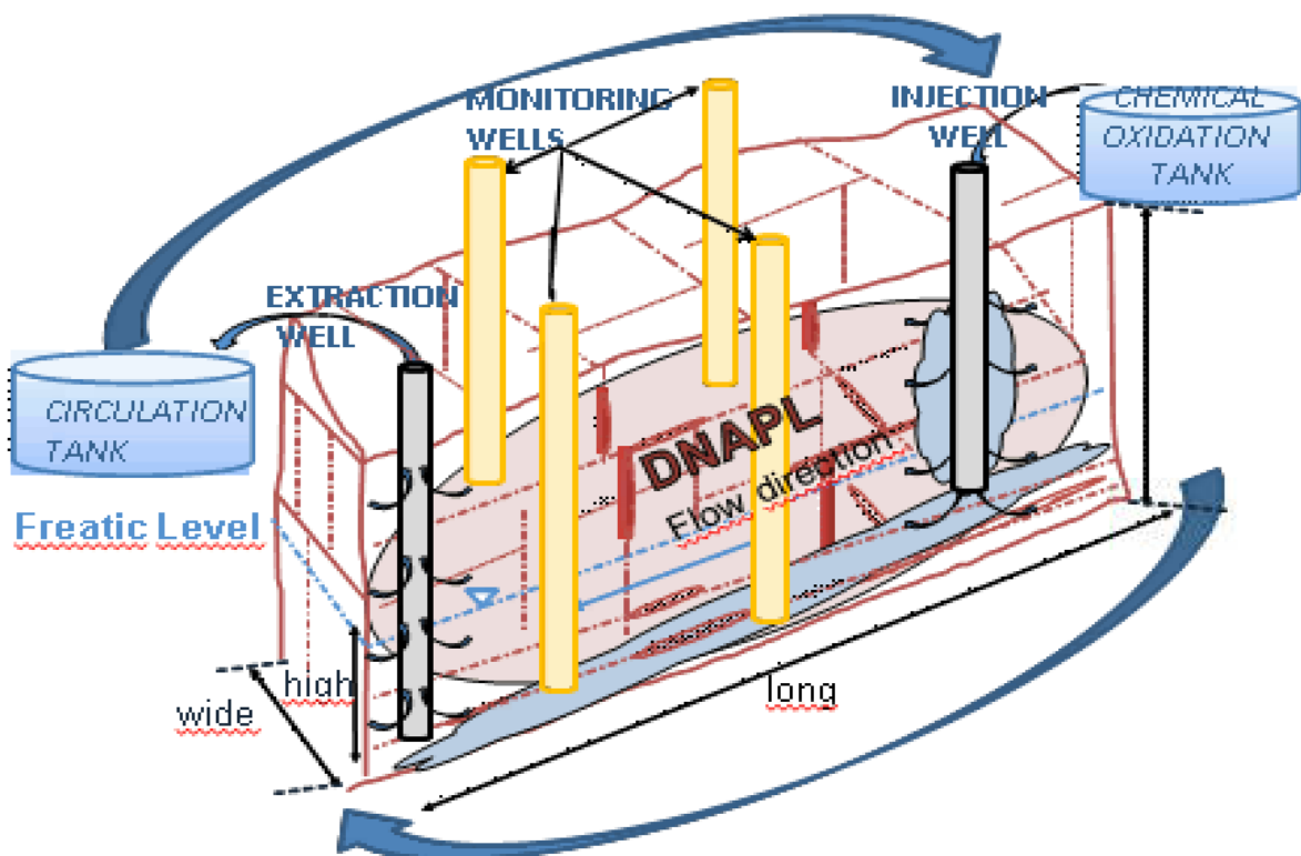
Rysunek 2.4- trójwymiarowy schemat recyrkulacji
