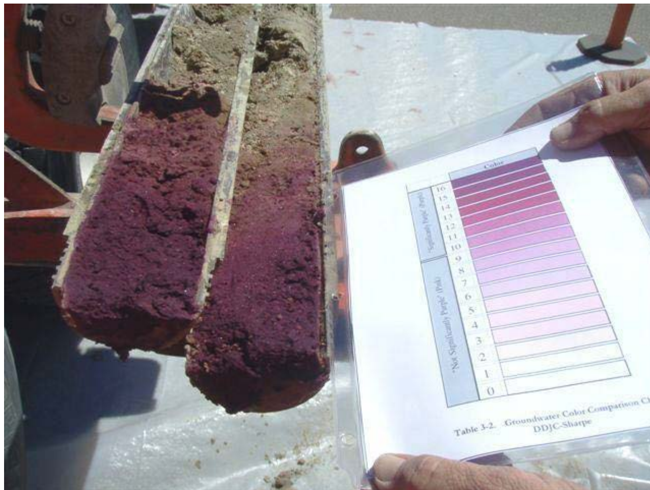
Rysunek 2.8- Przykład profilowania dyfuzji utleniacza w rdzeniu pyłu 90 dni po wprowadzeniu w szczeliny gruntowe preparatu z nadmanganianem potasu (zdjęcie dzięki życzliwości URS, Bures archive)
