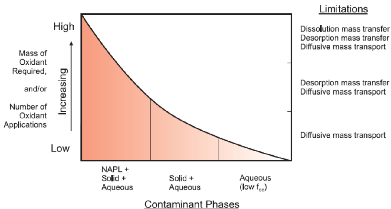
Rysunek 3.2- Wpływ faz zanieczyszczeń, możliwości i ograniczeń migracji na masę utleniacza i/lub liczbę zastosowań utleniacza potrzebnych do ISCO
