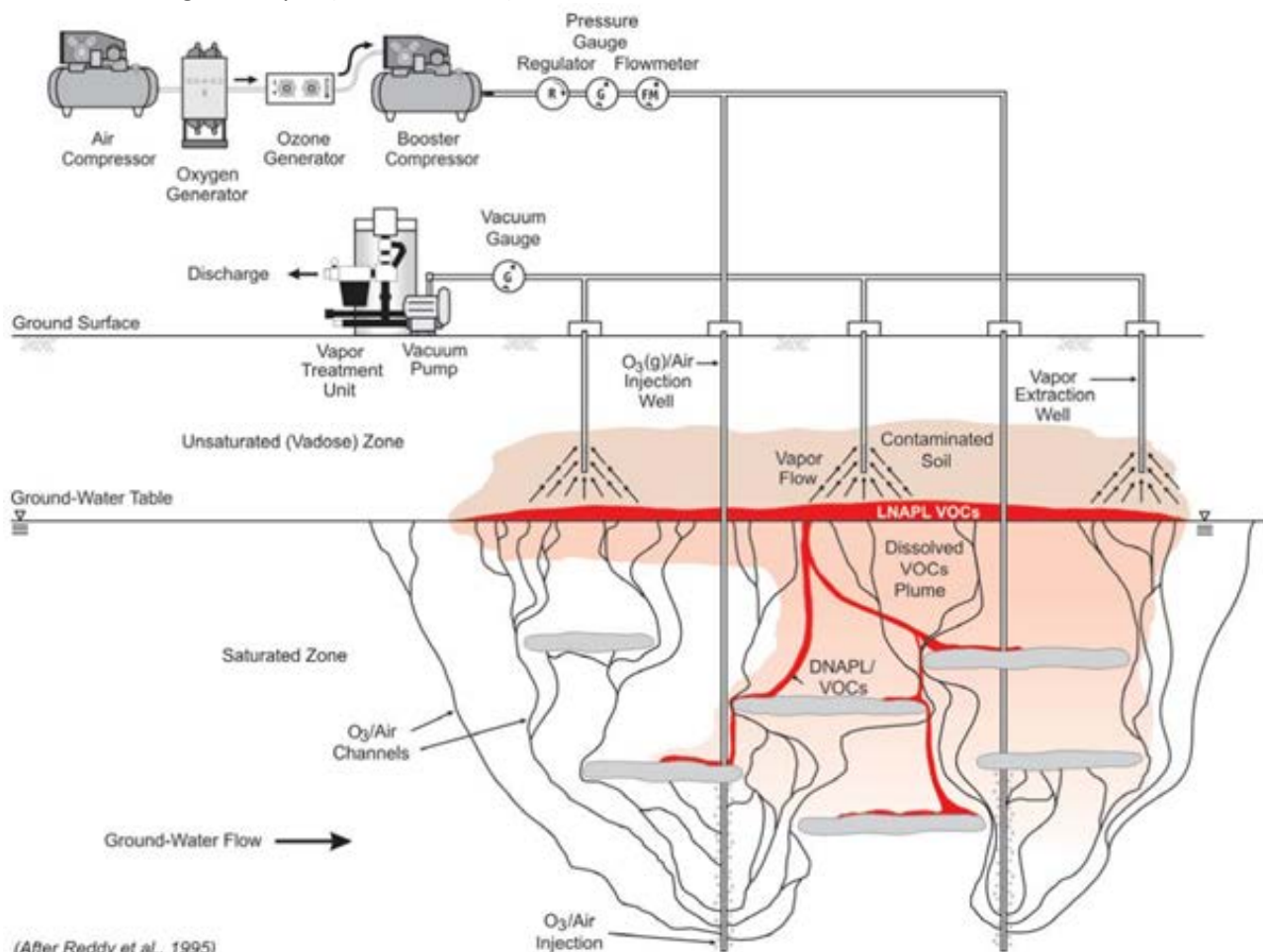
Rysunek 2.9- Ogólny model koncepcyjny ozonowania in situ w strefie saturacji z odciążeniem próżniowym z gruntu w celu wychwytywania emisji LZO i O 3
