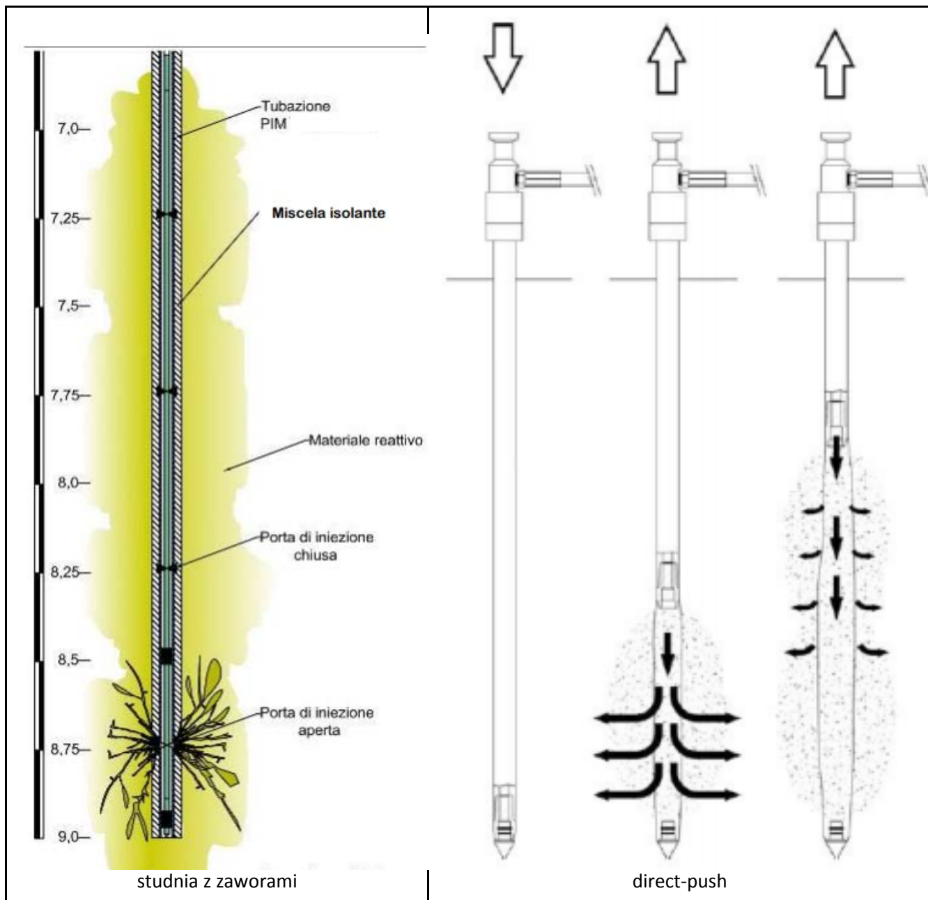
Rysunek 4.2 – Studnie z zaworami i wtłaczanie typu Direct-push
