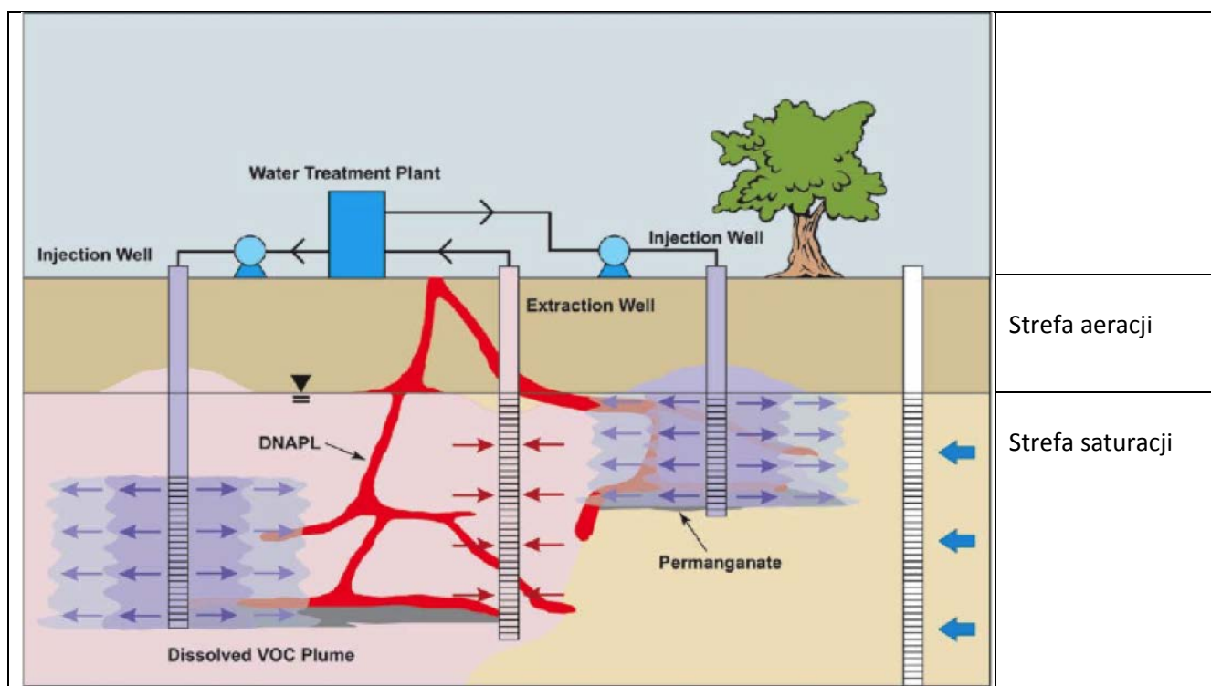
Rysunek 2.1- Schemat ISCO
