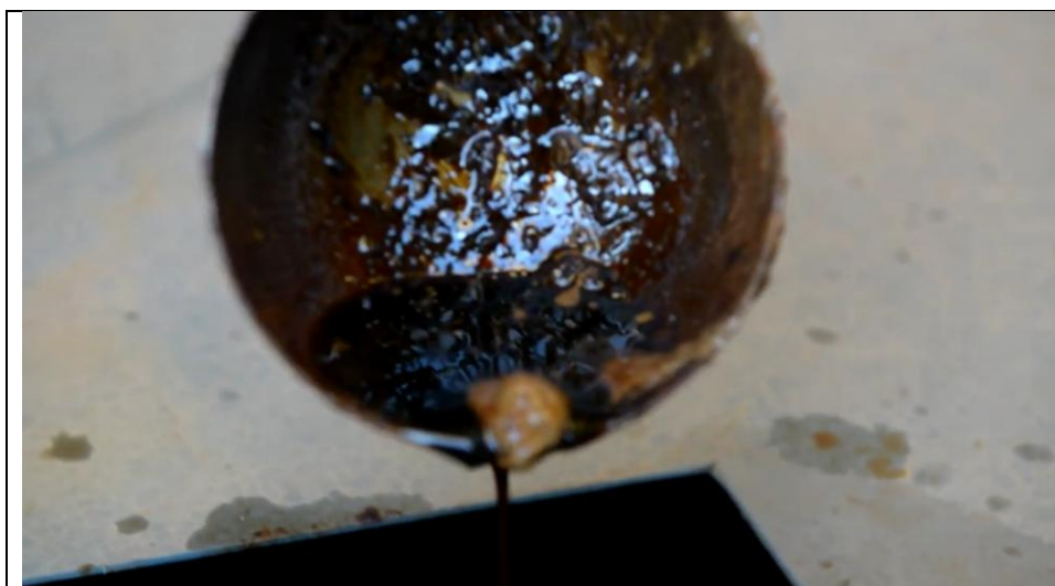
Figura 2.6- DNAPL
