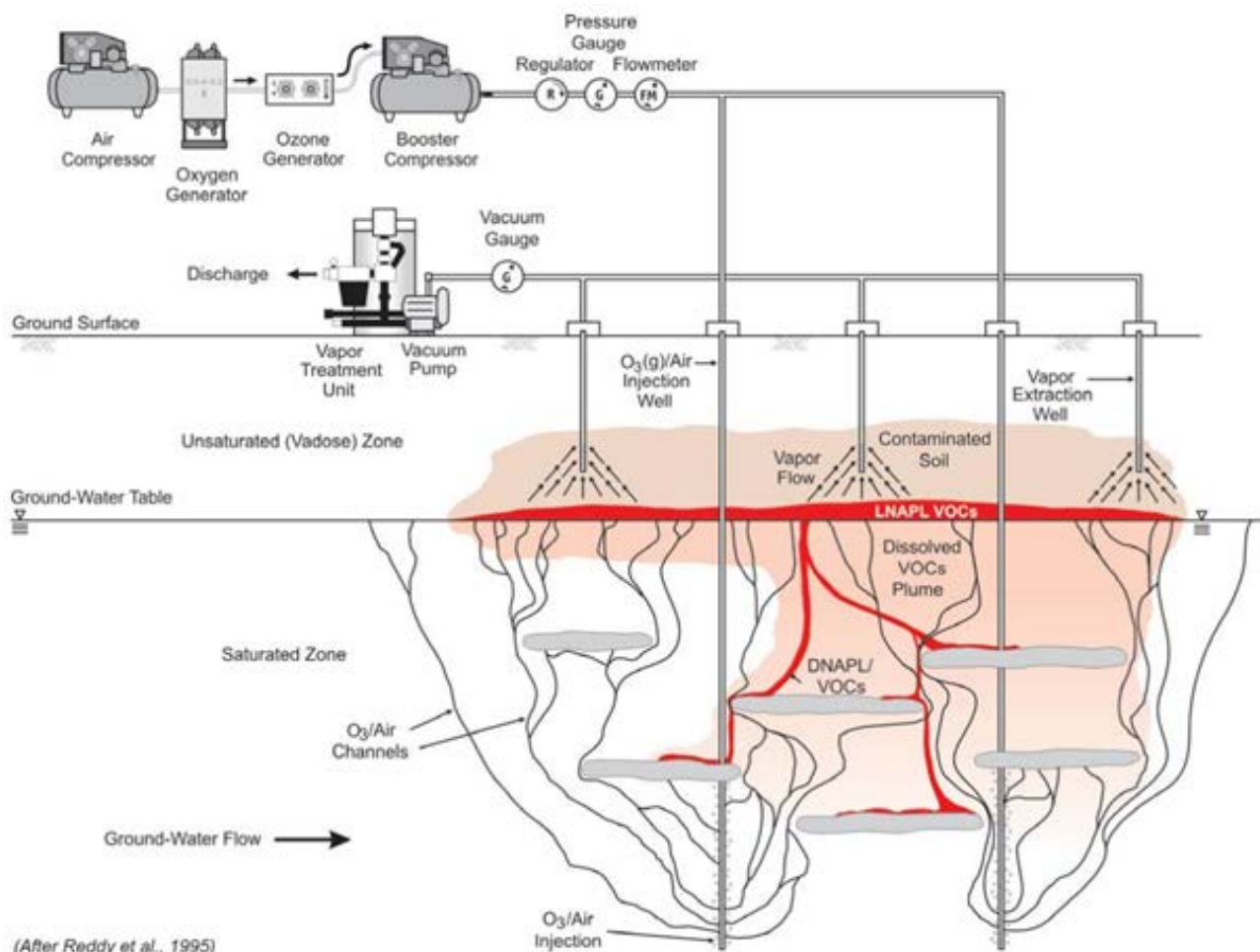
Σχήμα 2.9- Γενικό εννοιολογικό μοντέλο επιτόπιου οζονισμού στην κορεσμένη ζώνη με άντληση εδαφικού νερού για τη δέσμευση των πτητικών εκπομπών και του O 3 .
